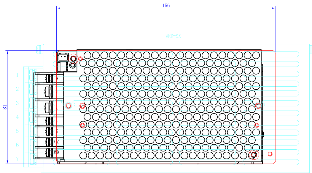
ESS100横置き アタッチメント1 WS-ES100-H1 ERD, WRD アルミ 板厚 5.0mm (ERD, WRDがM4仕様のため 他M3仕様)
