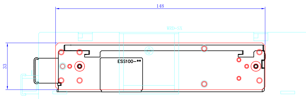
ESS100縦置き アタッチメント2 WS-ES100-T1 ERD, WRD, VTD アルミ 板厚 5.0mm (ERD, WRDがM4仕様のため 他M3仕様)
