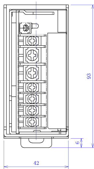
ESS150用DINレール対応取付金具外観図
