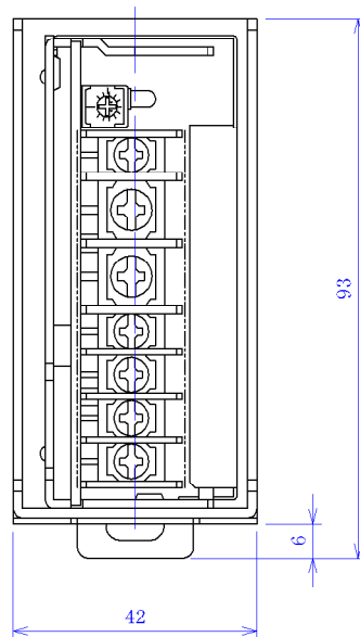
ESS100用DINレール対応取付金具外観図
