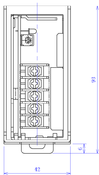
ESS50用D1Nレール対応取付金具外観図
