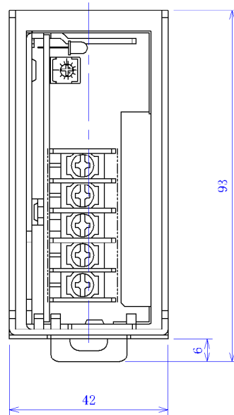
ES875用DINレール対応取付金具外観図
