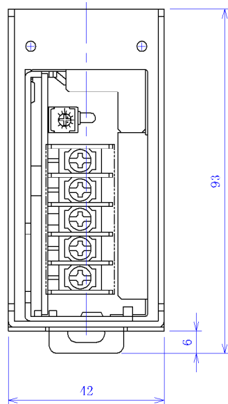
ESS30用DINレール対応取付金具外観図
