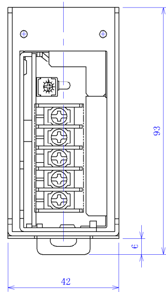
ESS15用DINレール対応取付金具外観図
