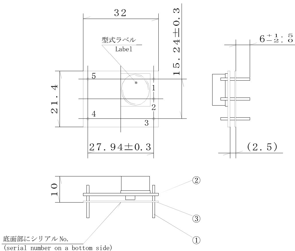
端子接続図 Pin Connection
