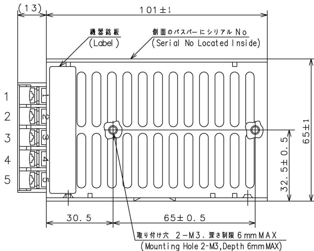
外觀・寸法図 Outline Drawing
