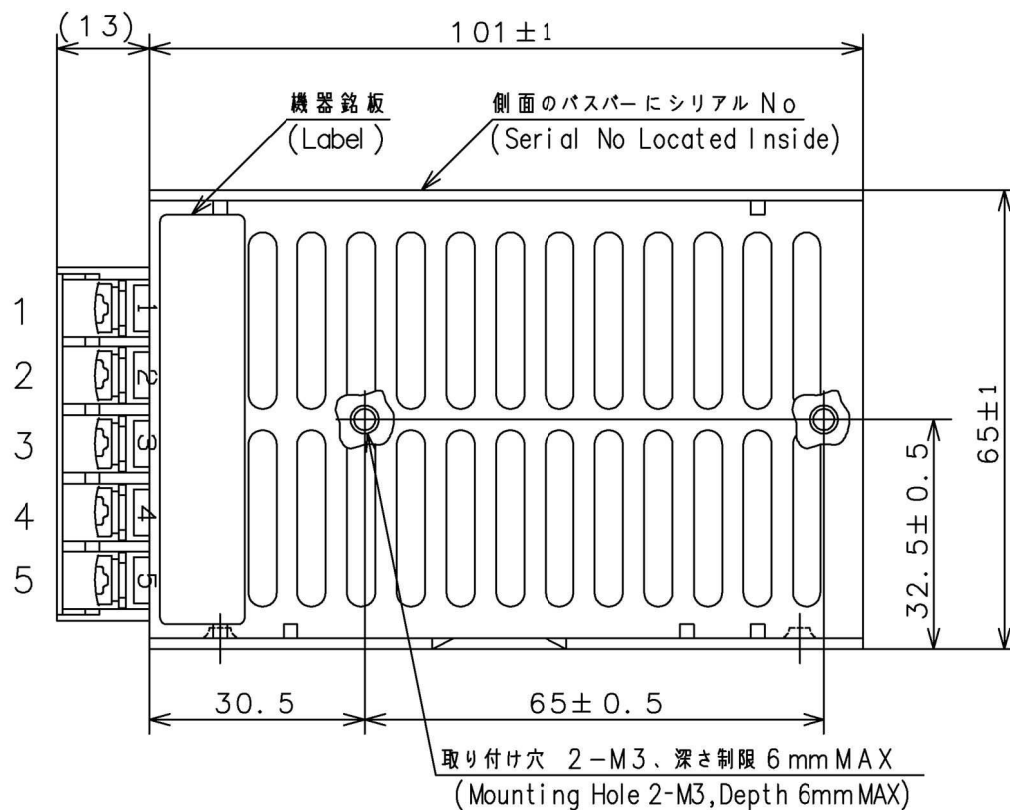
外觀・寸法図 Outline Drawing
