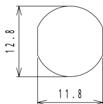
取付穴参考寸法 MOUNTING HOLE DIMENSION
