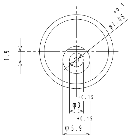
取付穴参考寸法 MOUNTING HOLE DIMENSION
