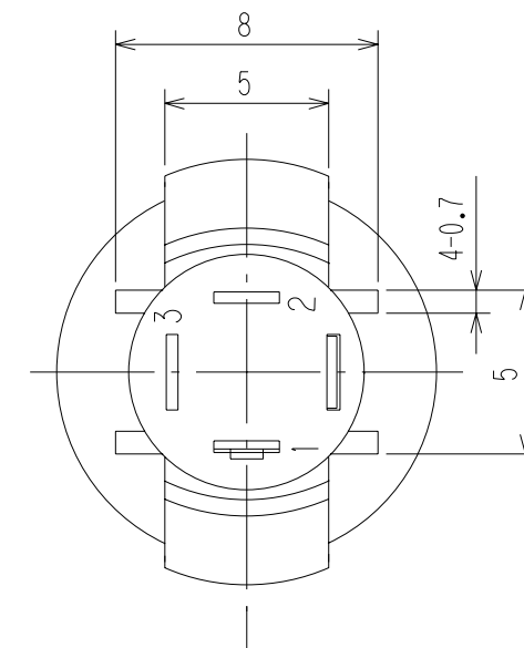
取付穴参考寸法 Mounting hole dimension
