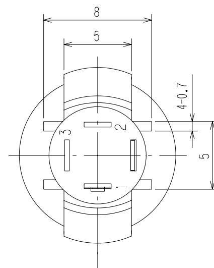
取付穴参考寸法 Mounting hole dimension
