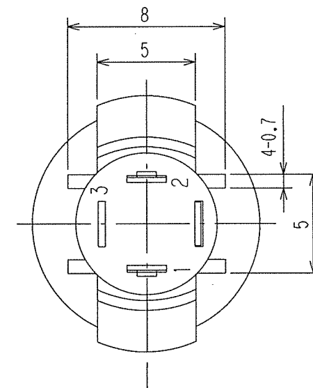
取付穴参考寸法 Mounting hole dimension
