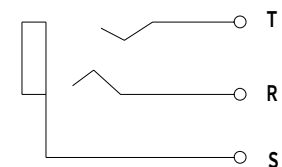
回路図
