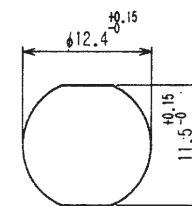
取付穴参考寸法
